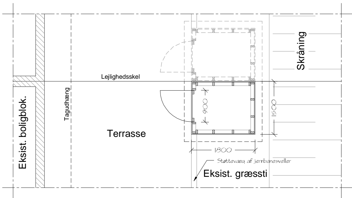
Plan, redskabsskur
