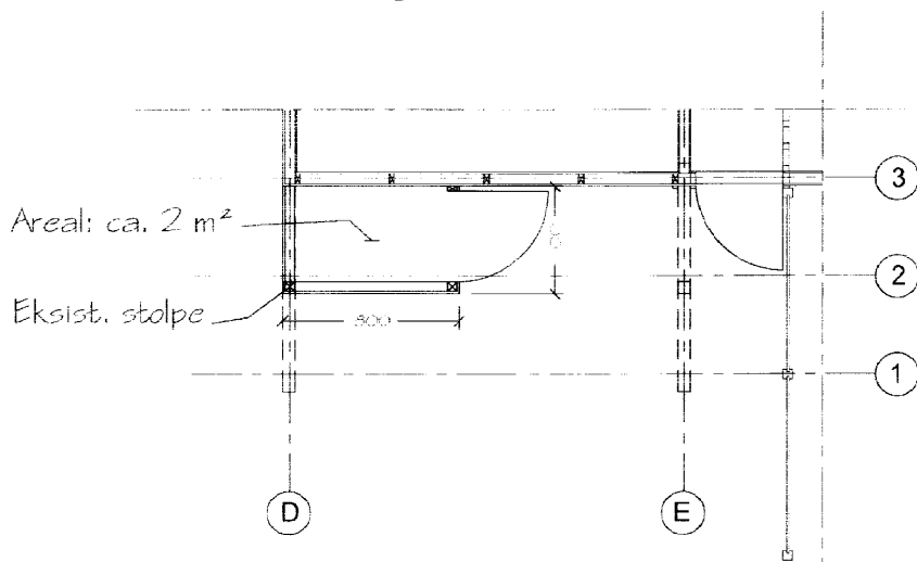
Stueplan
